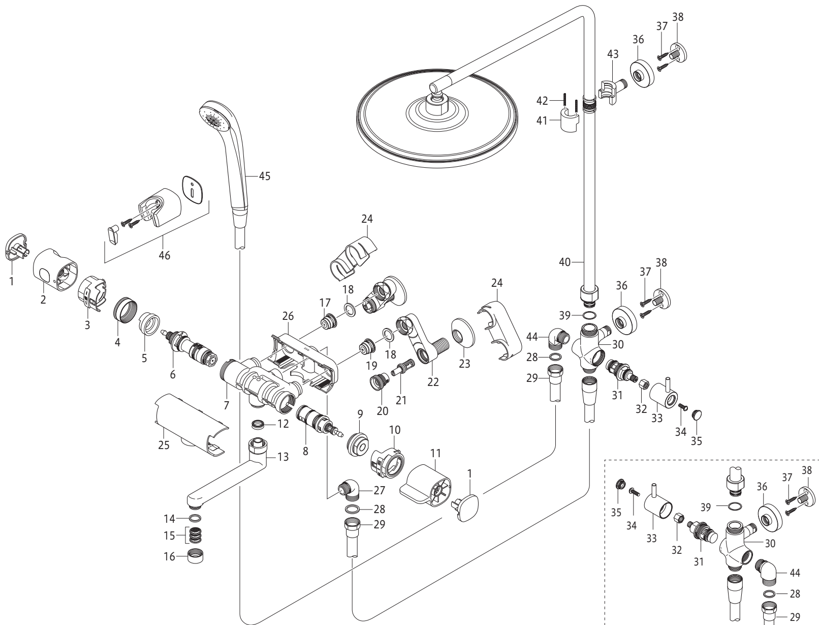
レバーハンドル左仕様
