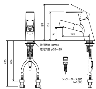
FSL150D(E)T(HS) <取付工具 KP5955 >
