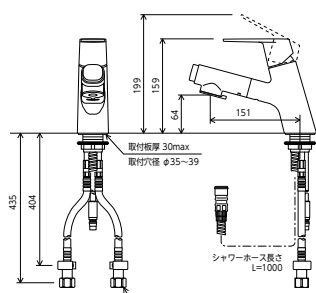
FSL150D(E)FT(HS) <取付工具 KP5955 >
