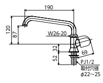
立形自在水栓 K16NDE [1/20] ¥6,650 (税込¥7,315) JIS プチエコ ■固定こま ■節水チップ内蔵型
