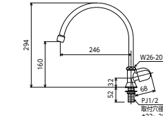
泡沫立形自在水栓 K16NDSLE [1/20] ¥8,290 (税込¥9,119) JIS 泡沫 プチエコ ■固定こま ■節水チップ内蔵型
