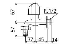
カップリング付横水栓 K4EJ [1/40] ¥6,400 (税込¥7,040) K4EZ [1/40] ¥5,700 (税込¥6,270) JIS 逆止 プチエコ ■固定こま ■節水チップ内蔵型 ■寒冷地用は逆止弁なし
