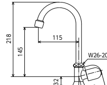
泡沫立形自在水栓 K16NDSFFE [1/20] ¥8,800 (税込¥9,680) JIS 泡沫 プチエコ ■固定こま ■節水チップ内蔵型
