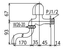
自在水栓 K3E [1/20] ¥6,000 (税込¥6,600) JIS プチエコ ■固定こま ■節水チップ内蔵型
