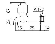
胴長横水栓 K2E [1/40] ¥5,800 (税込¥6,380) JIS プチエコ ■固定こま ■節水チップ内蔵型
