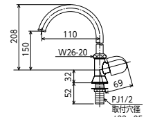
立形自在水栓 K16NDSSE [1/20] ¥7,250 (税込¥7,975) JIS プチエコ ■固定こま ■節水チップ内蔵型
