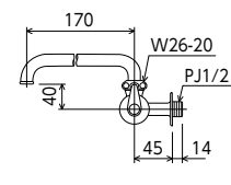
横形自在水栓 K10E [1/20] ¥6,300 (税込¥6,930) JIS プチエコ ■固定こま ■節水チップ内蔵型
