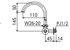
横形自在水栓 K10SSE [1/20] ¥6,500 (税込¥7,150) JIS プチエコ ■固定こま ■節水チップ内蔵型
