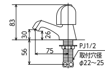
立水栓 K5E [1/40] ¥6,900 (税込¥7,590) JIS プチエコ ■固定こま ■節水チップ内蔵型
