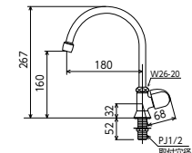
泡沫立形自在水栓 K16NDSFER2 [1/10] ¥9,430 (税込¥10,373) JIS 泡沫 プチエコ ■固定こま ■節水チップ内蔵型
