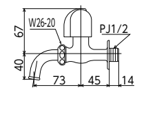
吐水口回転形水栓 K11E [1/40] ¥5,300 (税込¥5,830) JIS プチエコ ■固定こま ■節水チップ内蔵型
