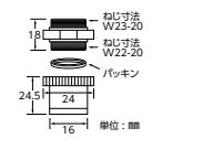
アダプターセット パイプ先端部取り付けタイプ PZ354 ¥1,610(税込¥1,771) [S] ■パイプ先端部の接続ジョイントです。
