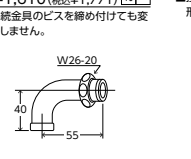
洗たく機用吐水口回転形水栓用ノズル13(1/2)用(W26-20) PZK04 ¥1,610(税込¥1,771) [I] ■接続金具のビスを締め付けても変形しません。
