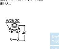
洗たく機用ノズル(直管)13(1/2)用 PZK97 ¥660(税込¥726) [I] ■接続金具のビスを締め付けても変形しません。
