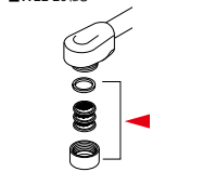
吐水口キャップセット 白 PZ511CP3 ¥1,180(税込¥1,298) [S] ■W22-20めねじ
