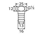
カラマイ、ナットセット13(1/2)用 PZK48 ¥660(税込¥726) [I]
