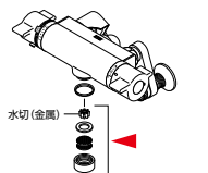
キャップセット(金属製水切) PZ422061S2 ¥1,650(税込¥1,815) [I] ■W26-20 ■水切が金属製のものが交換対象となります。
