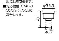
ワンタッチカバー(ホースクリップ付) PZ810 ¥1,330(税込¥1,463) [S] ■呼び13-20締め付け範囲13-22mm ■ホースを接続して、ワンタッチノズルに脱着できます。 ■対応機種:K34Bのワンタッチノズルに適合します。
