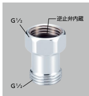
逆止弁付ジョイント(G1/2) Z411390SY ¥1,650(税込¥1,815) [1] [5]
