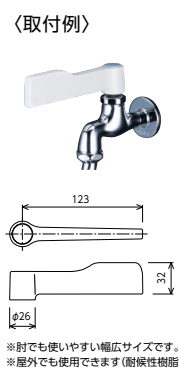
ワンタッチレバーハンドル PZS411 ホワイト ¥2,120(税込¥2,331) [5] [5]
