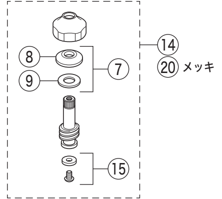
固定こま
